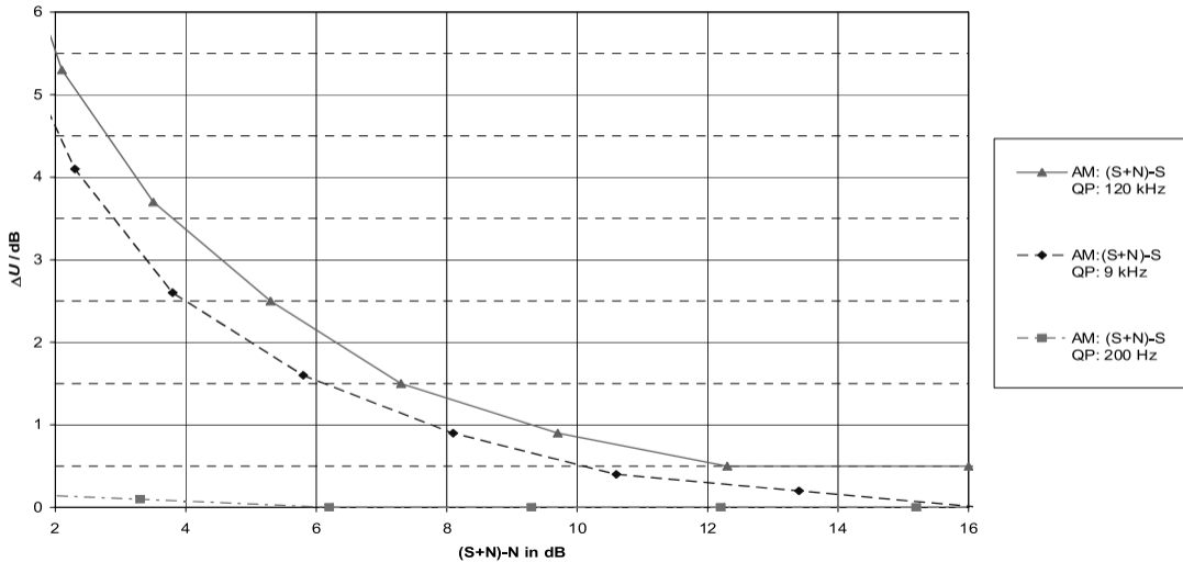
Differenz \Delta U des Messwerts abhängig von Verhältnis (S+N)/N für AM-modulierte Signale
