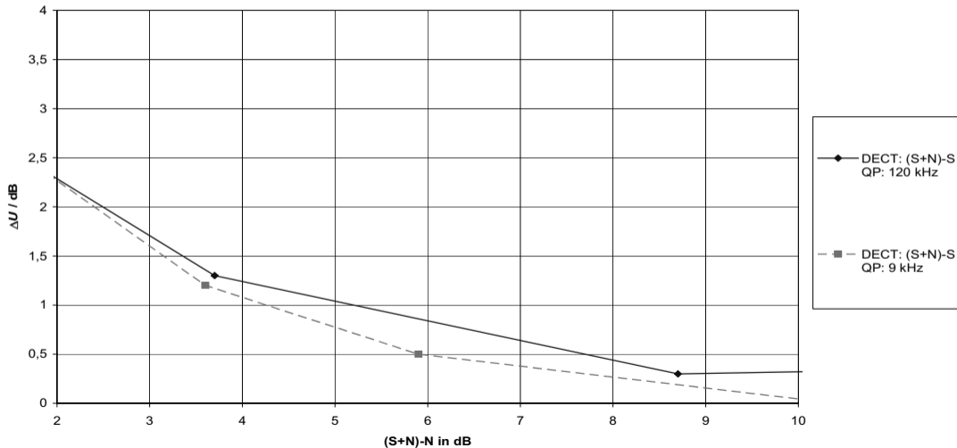
Differenz \Delta U des Messwerts abhängig von Verhältnis (S+N)/N für breitbandige digital modulierte Signale (z. B. DECT)
